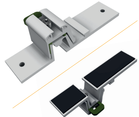
Mit vormontierten EPDM-Gummistreifen (UV-beständig)
