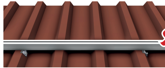
Unbedingt zu vermeiden ist die Montage von mehreren Trapez 2 an Seitenflanken, die in dieselbe Richtung zeigen.
